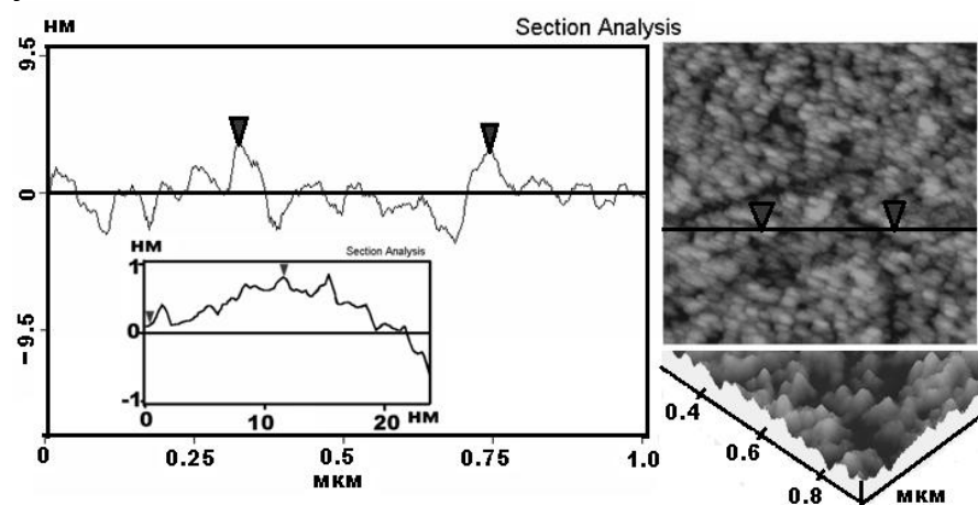
Рис. 1. Распределение размеров неоднородностей в плоскости образца № 7 (на вставке: отрезок кривой в увеличенном масштабе) и вид сверху и сбоку на поверхности образца.
