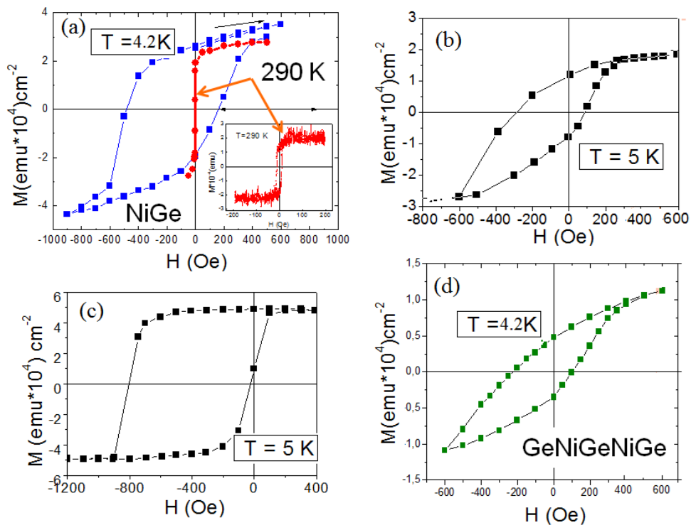
Рис. 10. Низкотемпературные полевые зависимости намагненности для двухслойных пленок Ni/Ge (a–c) и пятислойной пленки (d). Магнитное поле параллельно плоскости пленок. Вставка (a): петля гистерезиса при 290 К.
