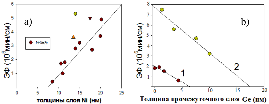
Рис. 8. (а) Удельный ЭФ для двухслойных пленок в поле насыщения образцов, приведенных в табл. 1, и (б) – удельный ЭФ для двух серий пятислойных пленок, табл. 2, с суммарной толщиной Ni ~22 нм (1) и ~ 32 нм (2) в поле насыщения.
