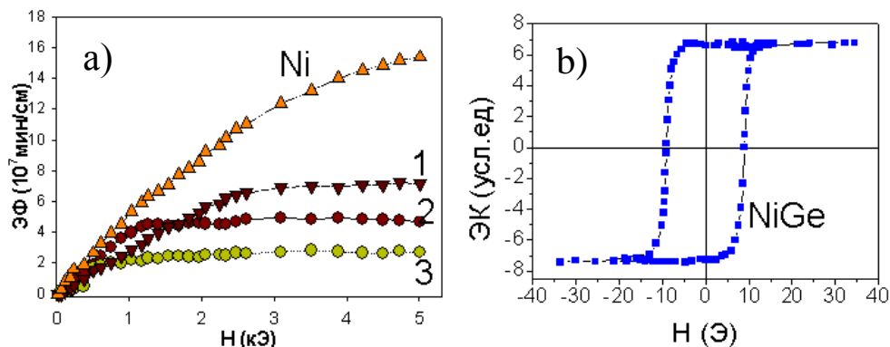
Рис. 7. (а) – полевые зависимости ЭФ для образцов Ni (20.4 нм) и № 12, 8, 5 (кривые 1–3 соответственно), \lambda = 900 нм, и (b) – эффект Керра для образца № 12, \lambda = 632.8 нм.
