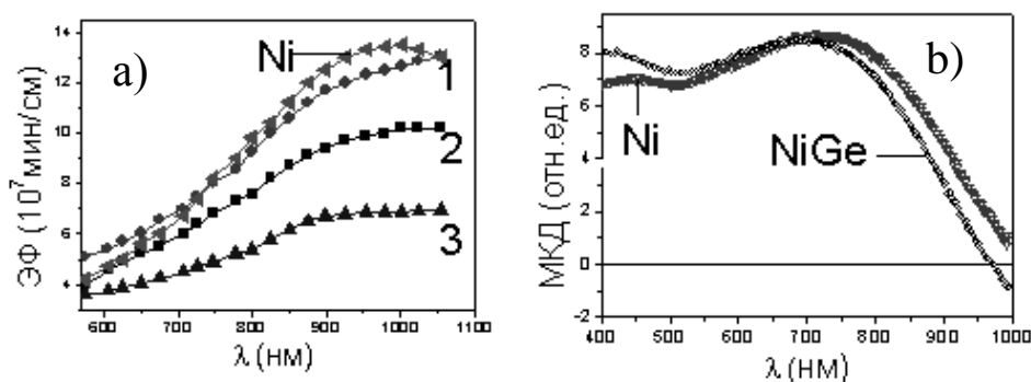
Рис. 6. (а) – спектры ЭФ в поле 1,3 кЭ для образцов Ni (17 нм) и № 22, 21, 24 (кривые 1–3 соответственно) и (b) – спектры МКД пленки Ni (20.4 нм) и образца № 14.
