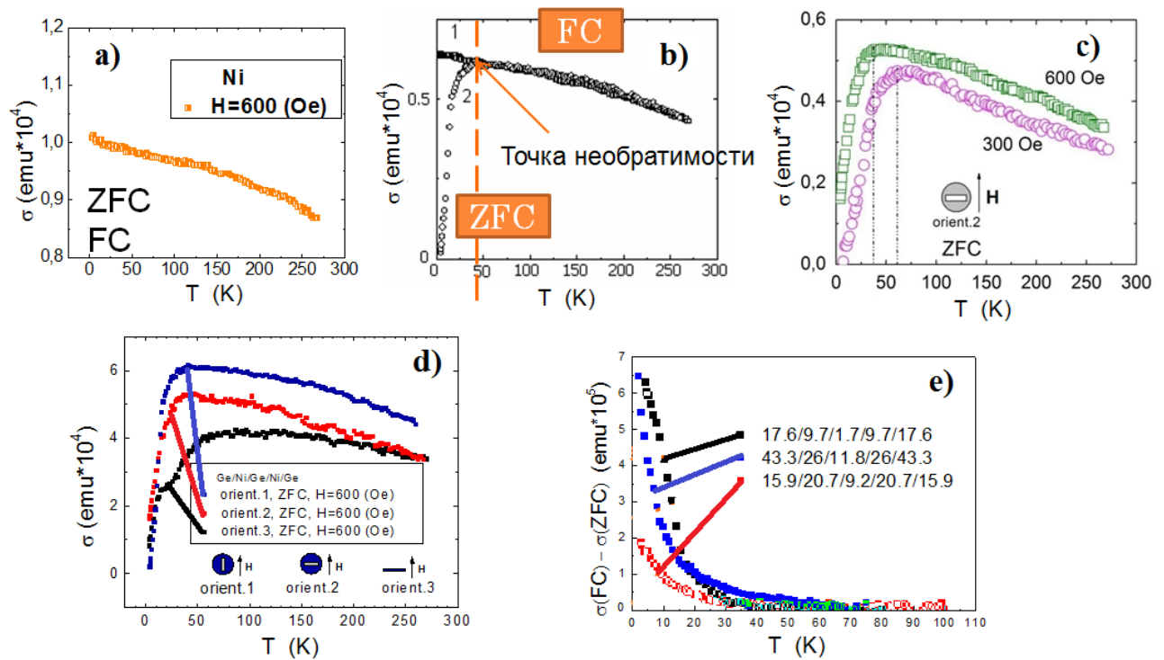
Рис. 9. Температурные зависимости намагненности для режимов охлаждения FC и ZFC пленки Ni (a) и двухслойной пленки, H = 600 Э (b); ZFC кривые двухслойной пленки для полей 300 и 600 Э (c) и трех различных ориентаций образца в поле 600 Э (d); разности FC и ZFC кривых для трех пятислойных образцов.
